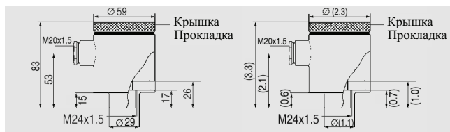
Соединительная головка, форма В-VA, класс защиты IP65, из нерж. стали, с винтовой крышкой, размеры в мм (дюймах)
