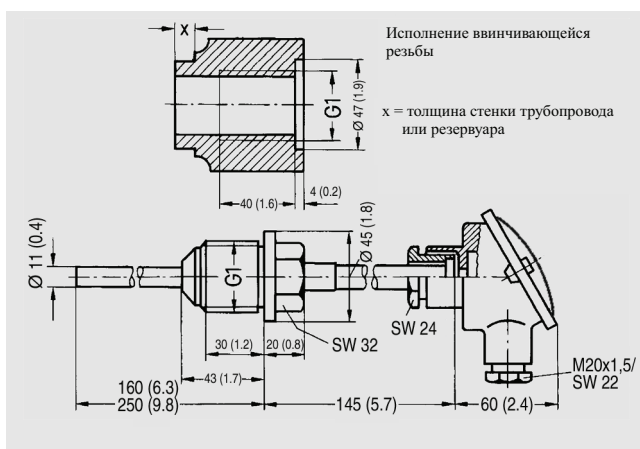
Ввинчивающийся термометр сопротивления высокого давления с соединительной головкой с консолью, размеры в мм (дюймах)
